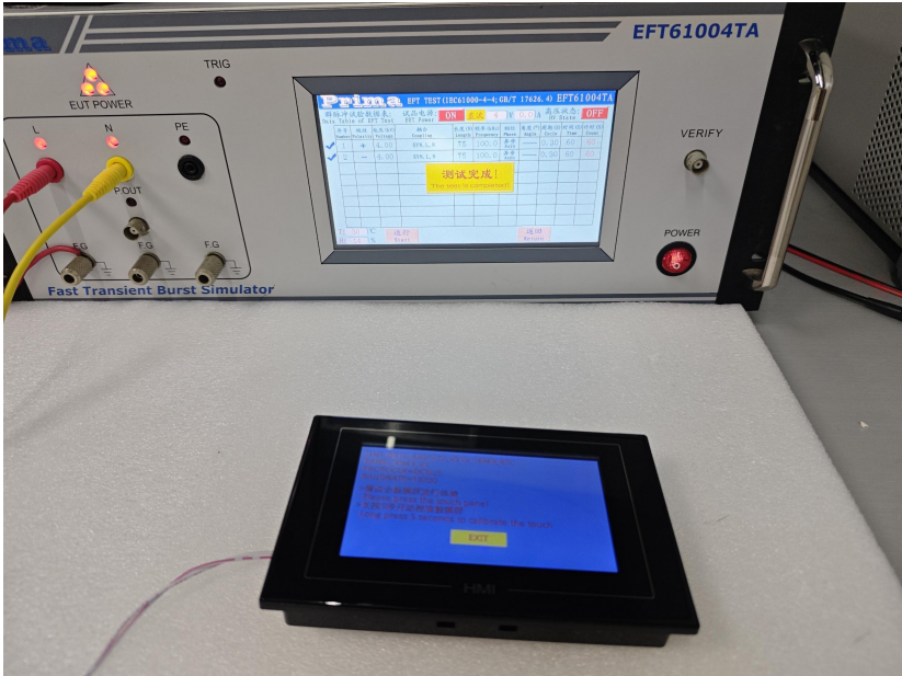
图 6-4 群脉冲测试图
