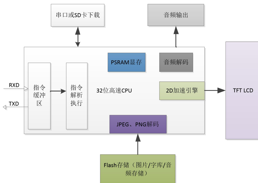
图 3-1 DB 系列串口屏内部结构图
