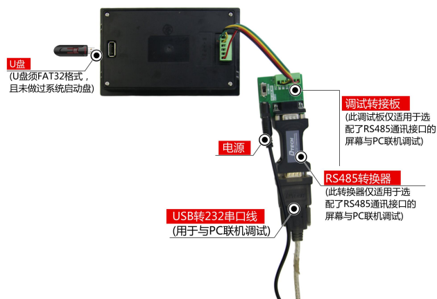
图 1-5 RS485 调试工具图
