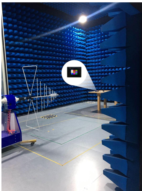
图 6-5 辐射测试图
