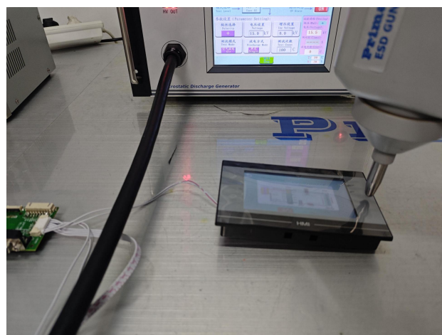
图 6-2 ESD 测试图
